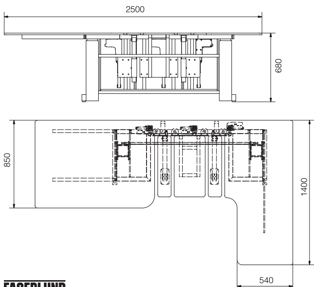
Individuelle justeringshøjder.
